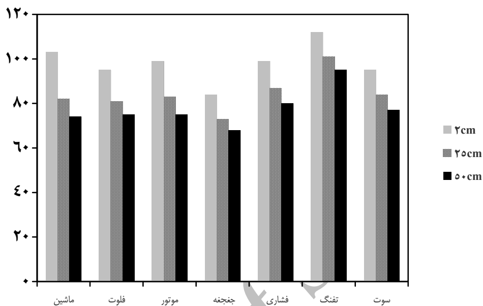
نمودار 1- شدت نویز در اسباب بازی های دارای نویز مداوم
