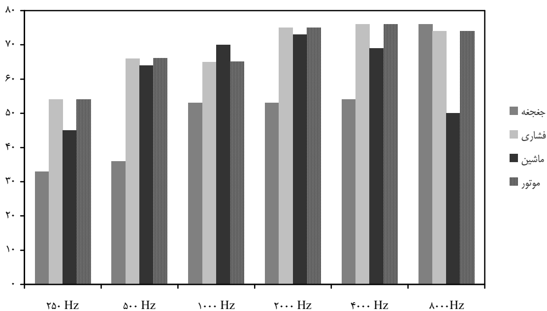
نمودار 3- تحلیل فرکانسی در برخی از اسباب بازی ها
